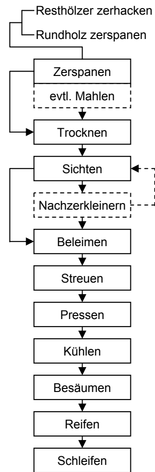
Abbildung 2-5: Arbeitsablauf Spanplattenherstellung
