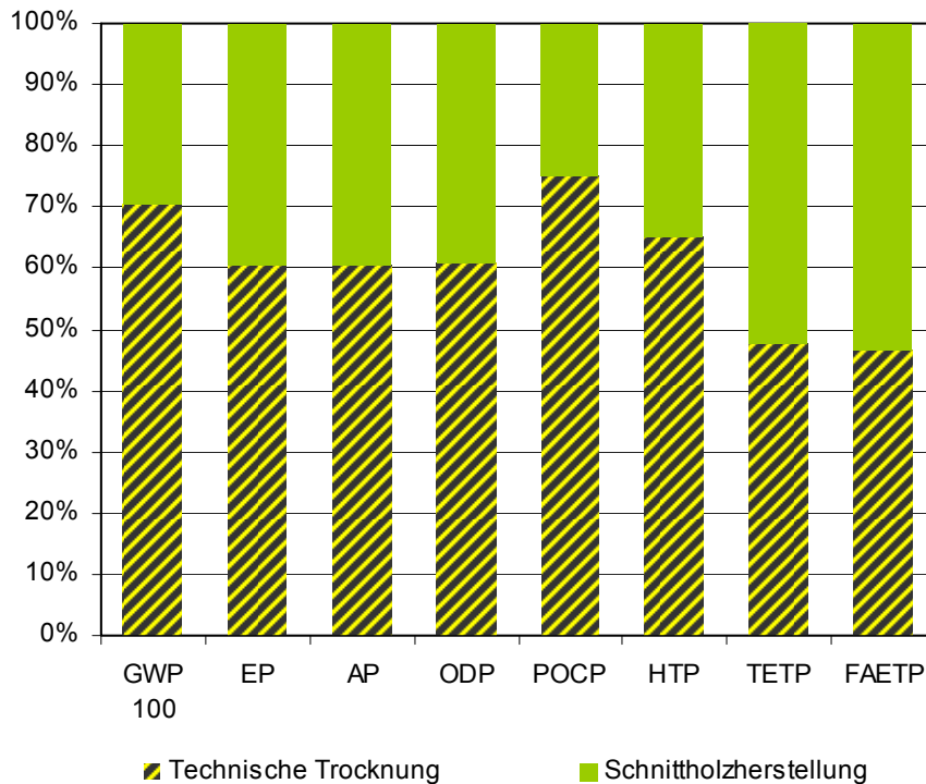
Abbildung 2-14: Anteil der technischen Trocknung an den Umwelteinträgen von getrocknetem Schnittholz nach Wirkungskategorien
