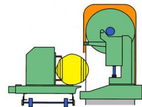
Abbildung 2-4: Band- säge (Linck, 2006)
