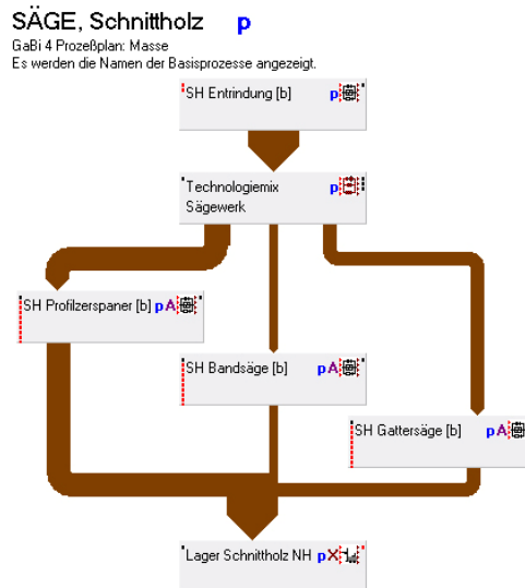
Abbildung 2-10: Modellierung der Einschnittechnologie im Modul Sägewerk
