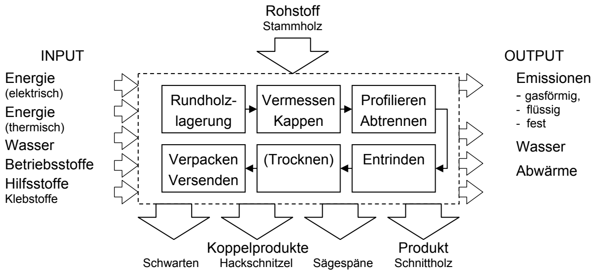
Abbildung 2-7: Der Bilanzraum des Moduls Schnittholzherstellung
