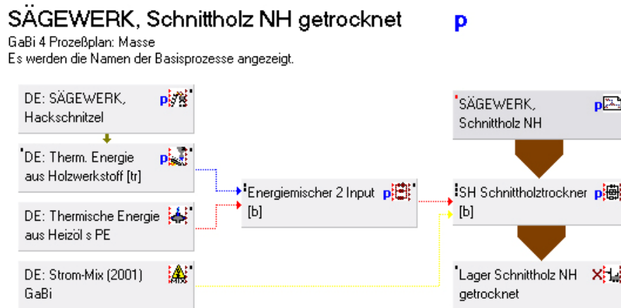
Abbildung 2-12: Modellierung des Trocknungsprozesses
