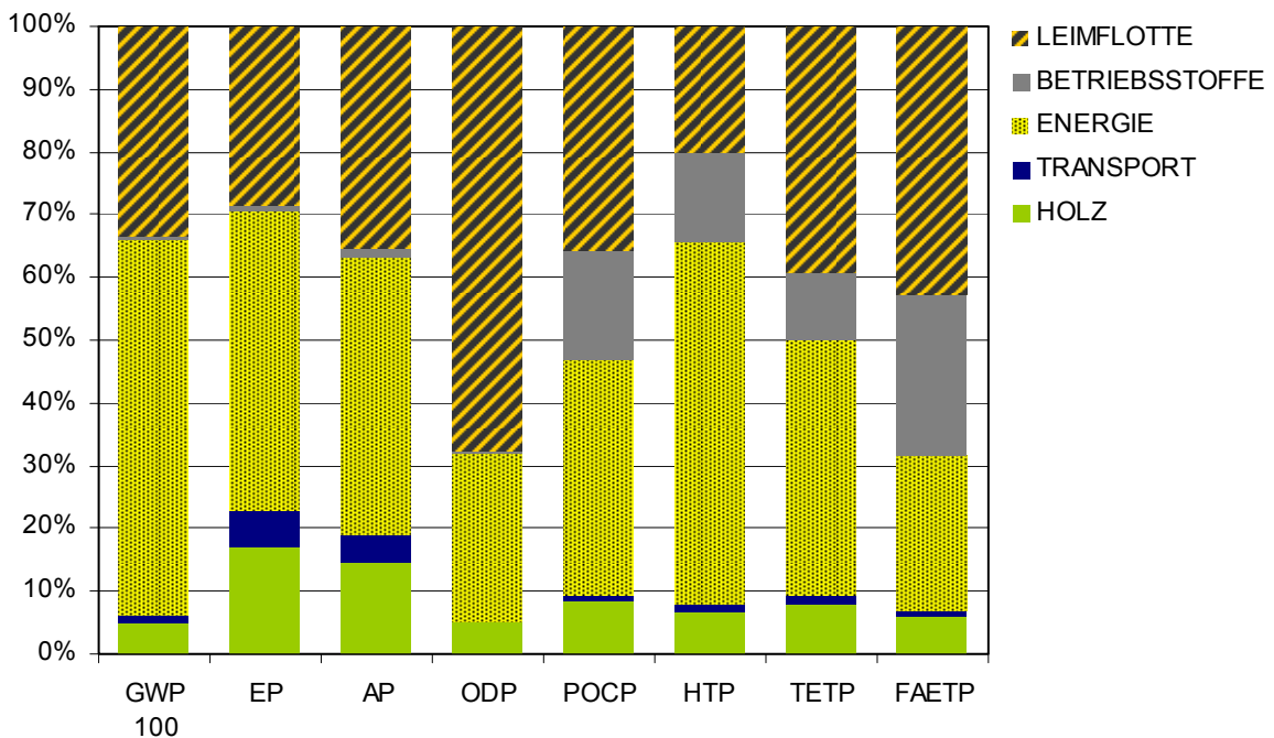
Abbildung 2-16: Ergebnisse der Ökobilanz für Spanplatte P7
