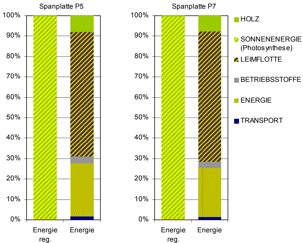
Abbildung 2-17: Primärenergieaufwand für die Produktion von Spanplatten P5 und P7
