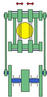
Abbildung 2-3: Vollgatter (Linck, 2006)
