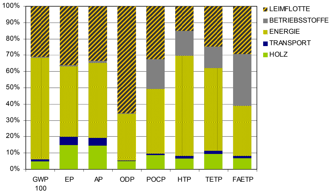
Abbildung 2-15: Ergebnisse der Ökobilanz für Spanplatte P5
