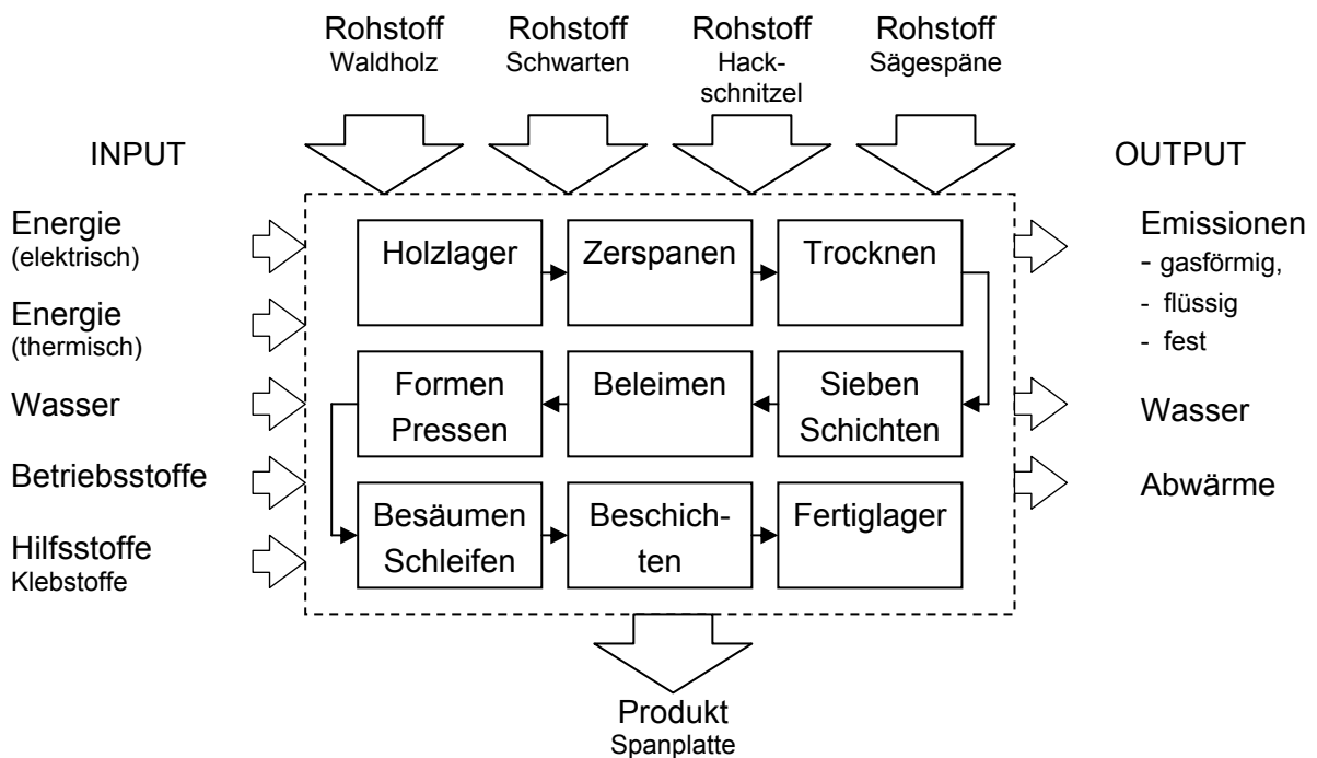
Abbildung 2-8: Der Bilanzraum des Moduls Spanplattenherstellung
