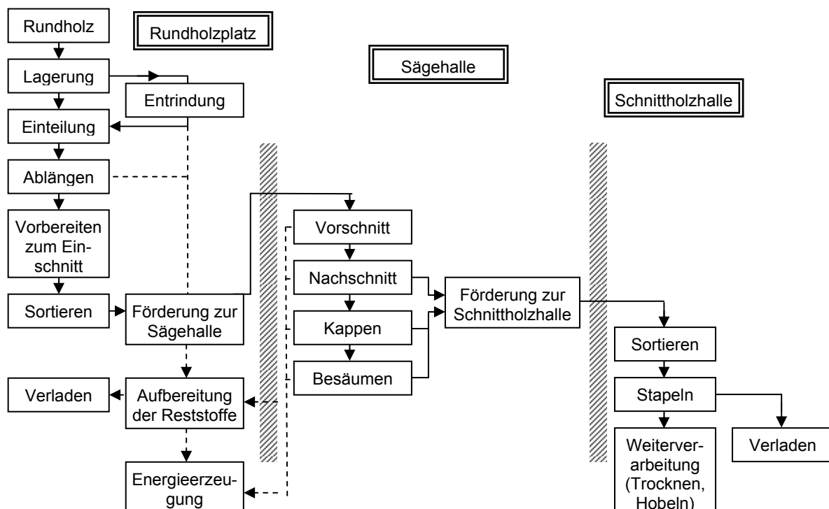
Abbildung 2-1: Schematischer Arbeitsablauf im Sägewerk
